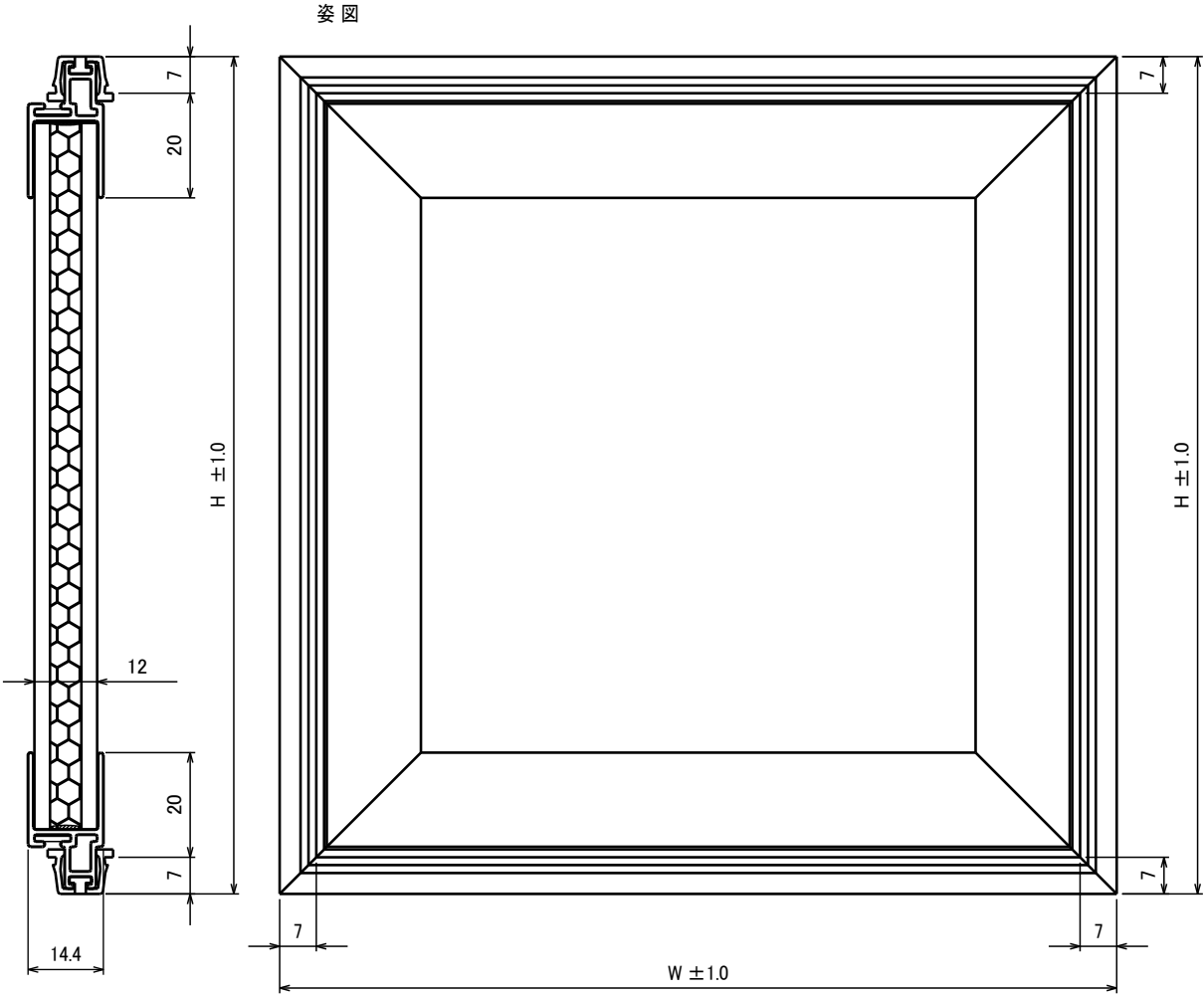
ZAA025-BC05D ダンプネル(単板アタッチメント付) 商品図
