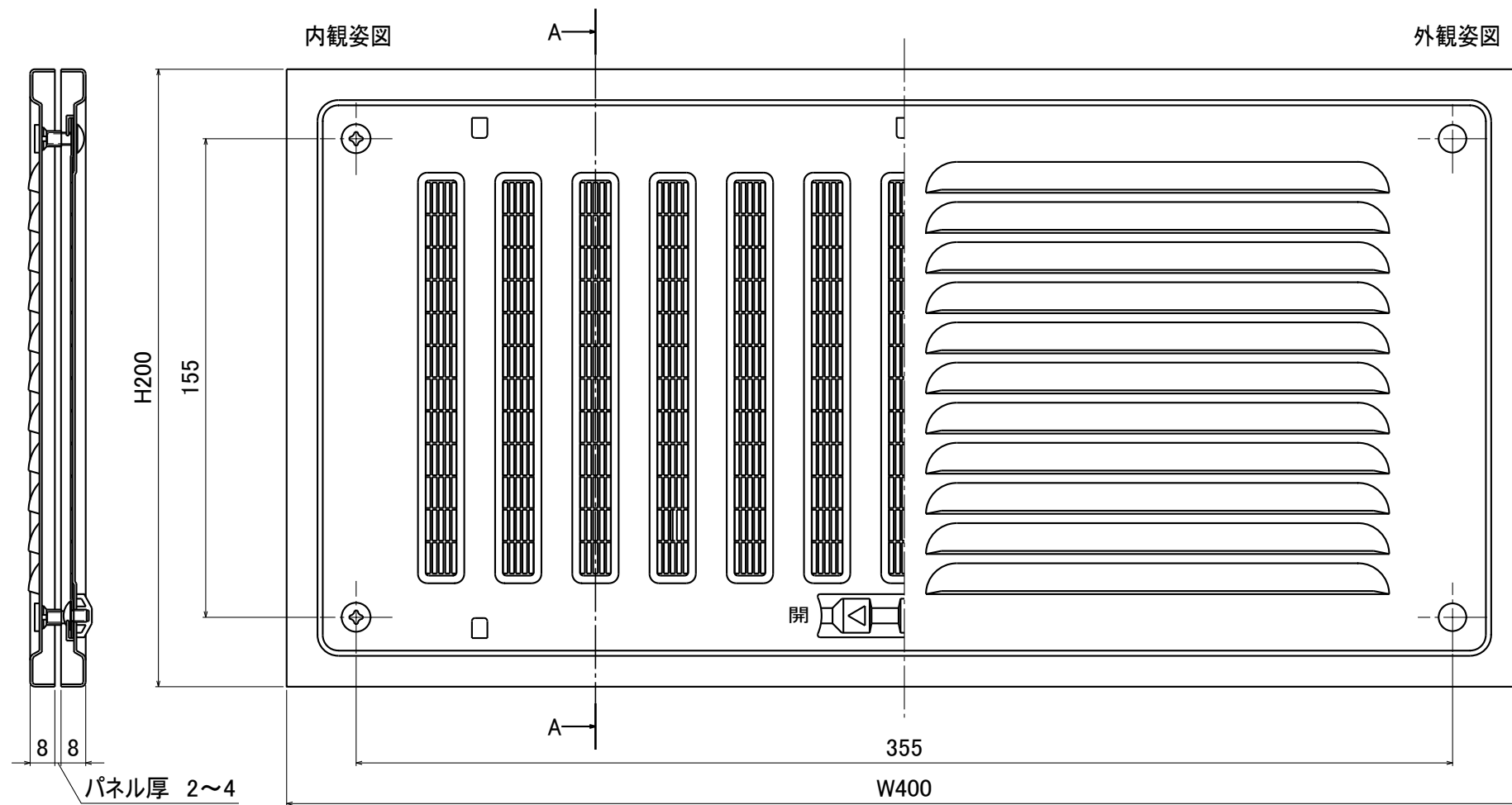
A-A断面図
