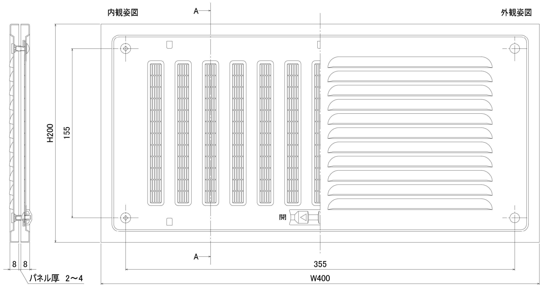
A-A断面図
