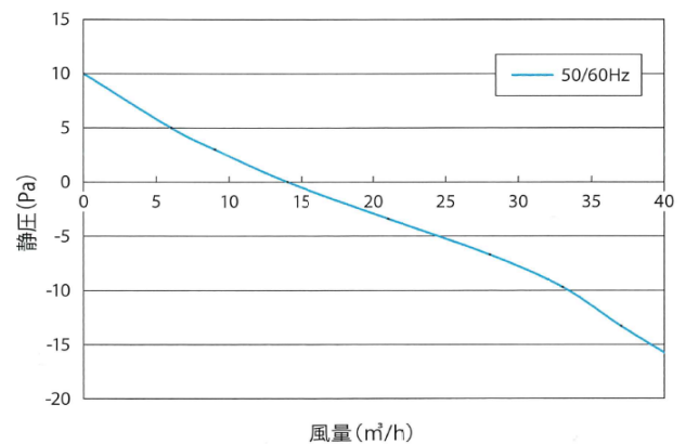
PQ曲線図
