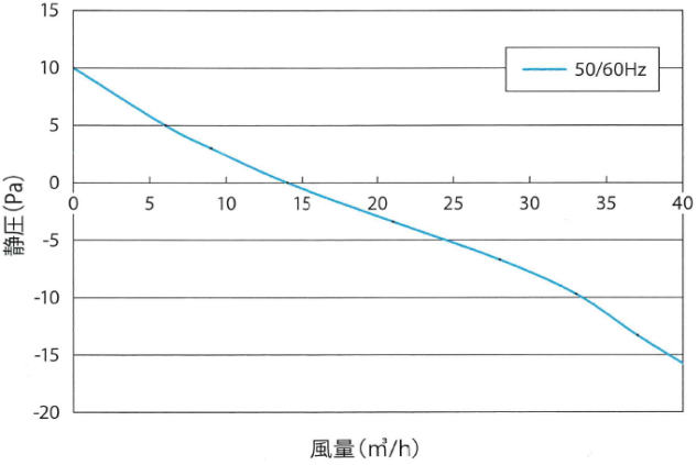
PQ曲線図
