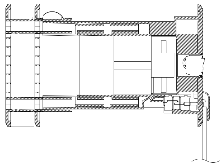
B-B断面図
