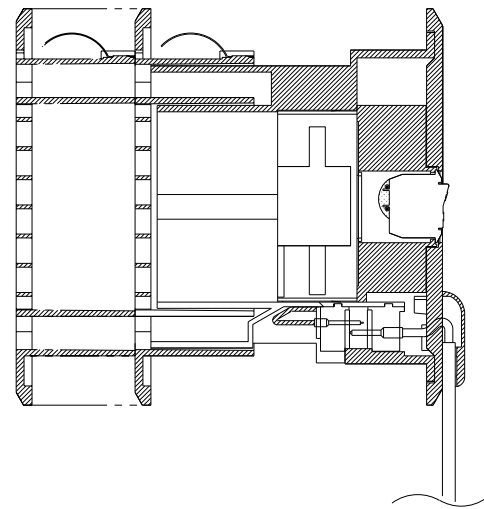
B-B断面图
