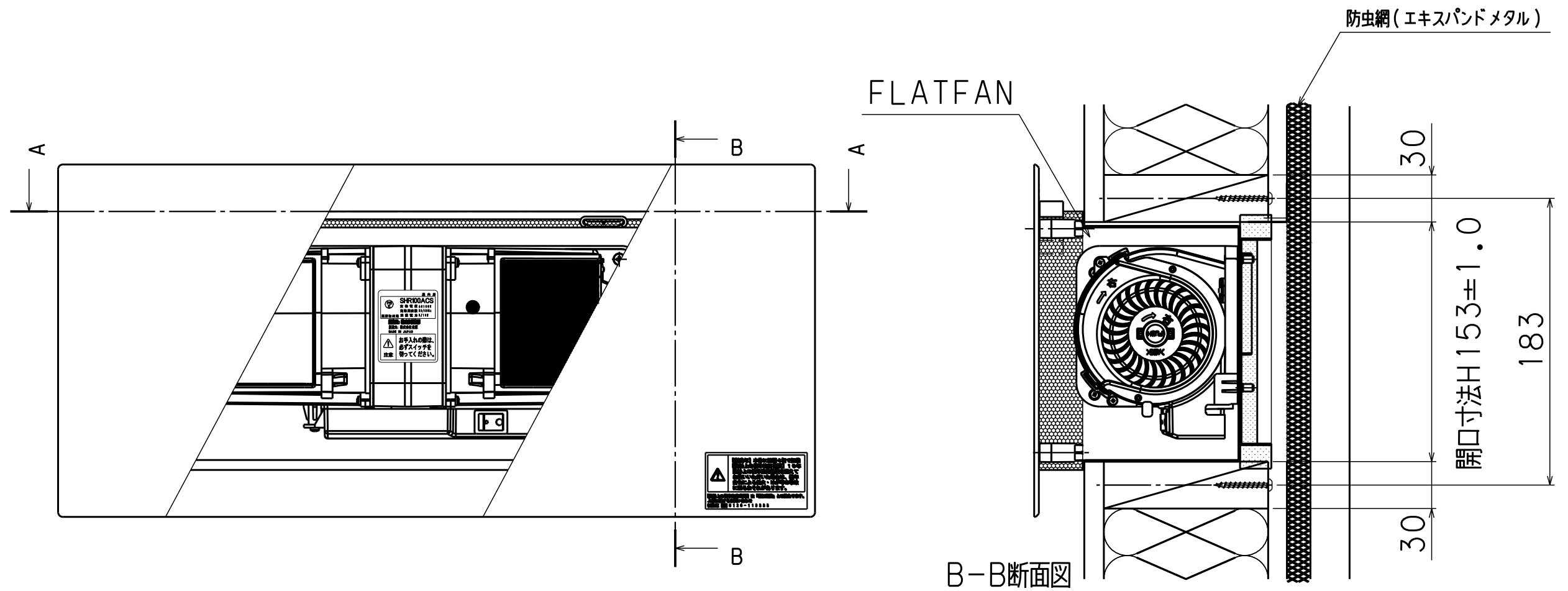
ZAA187-FB03 FLATFAN 横胴縁納まり図 (柱105)
