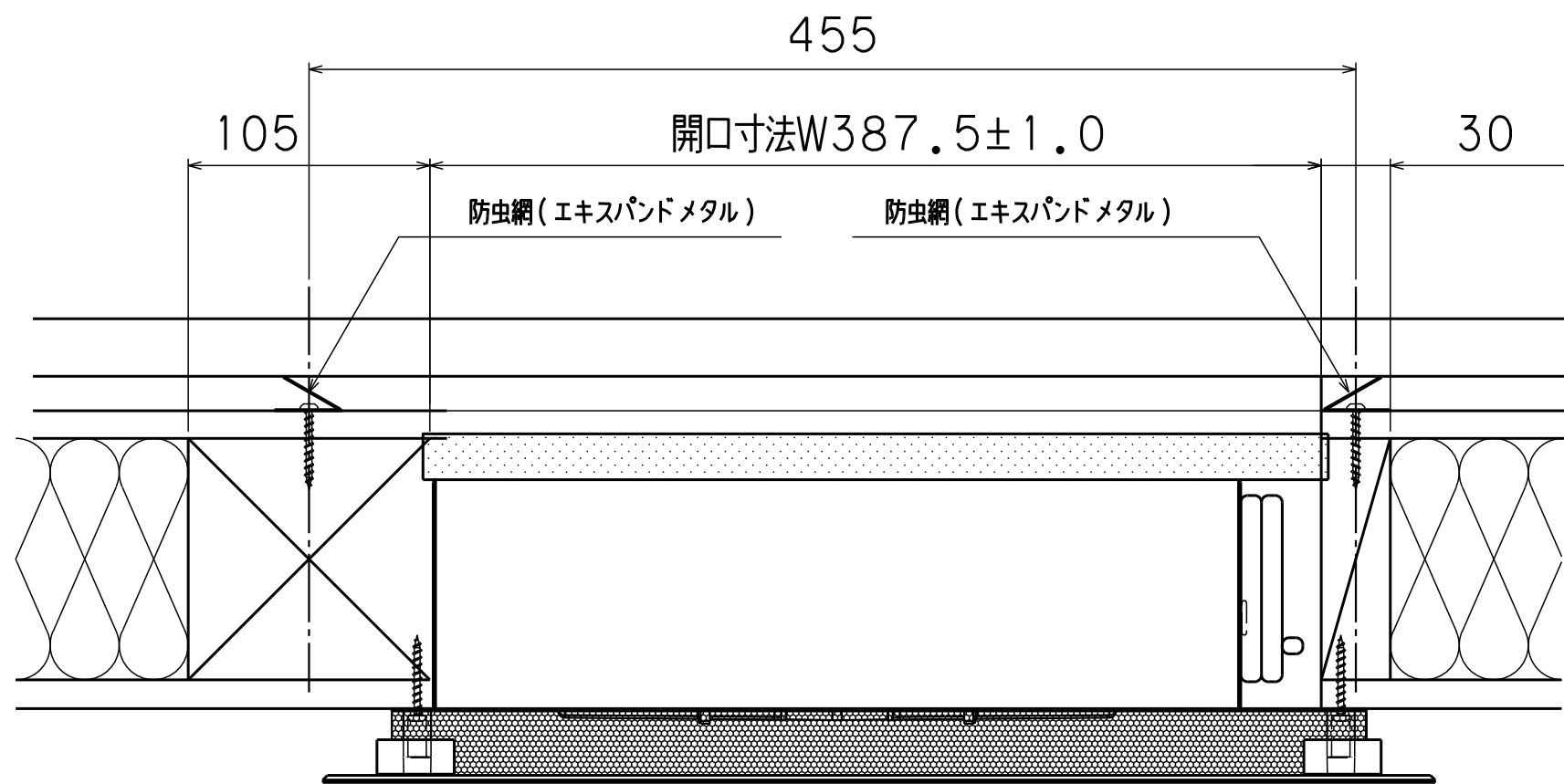
A-A断面図
