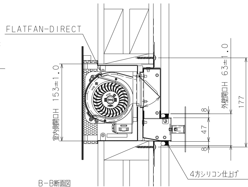
ZAA194-FB03 FLATFAN-DIRECT 2*4納まり図
