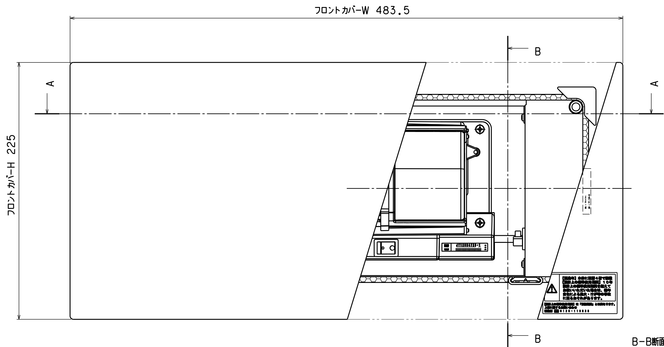
A-A断面図
