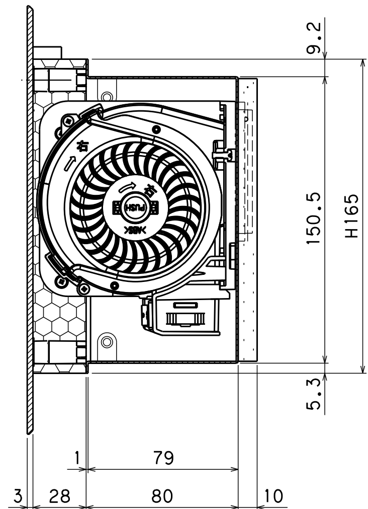
B-B断面図
