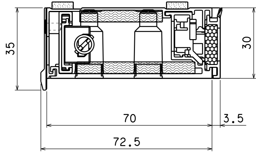
A-A断面図
