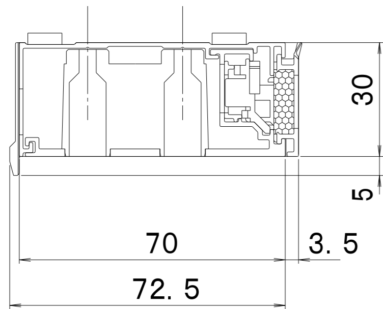
A-A断面図
