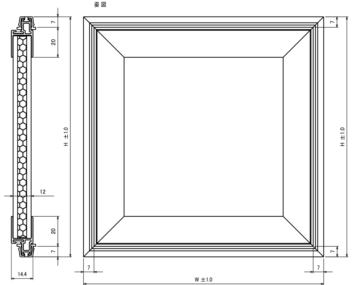
ZAA025-BC05C ダンパネル(単板アタッチメント付) 商品図
