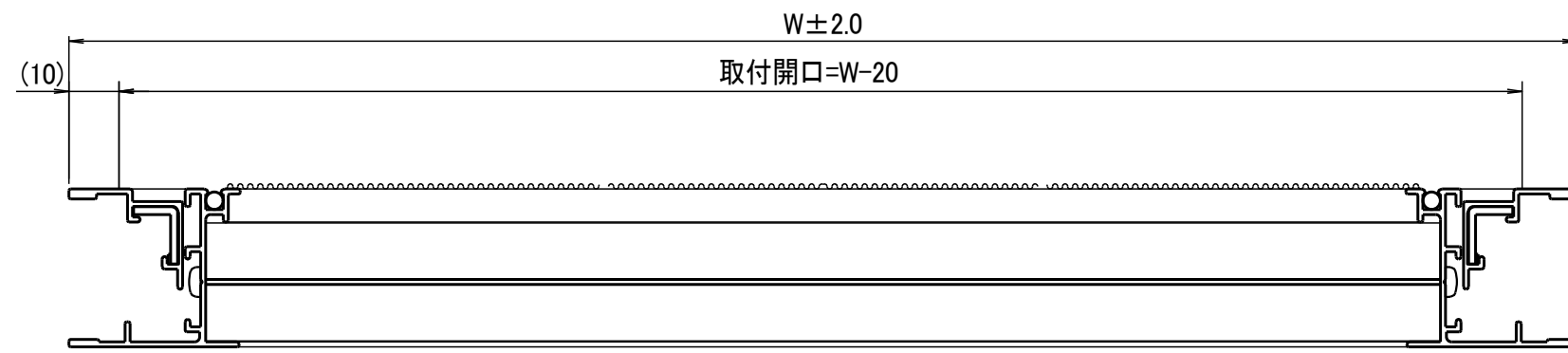
A-A断面図
