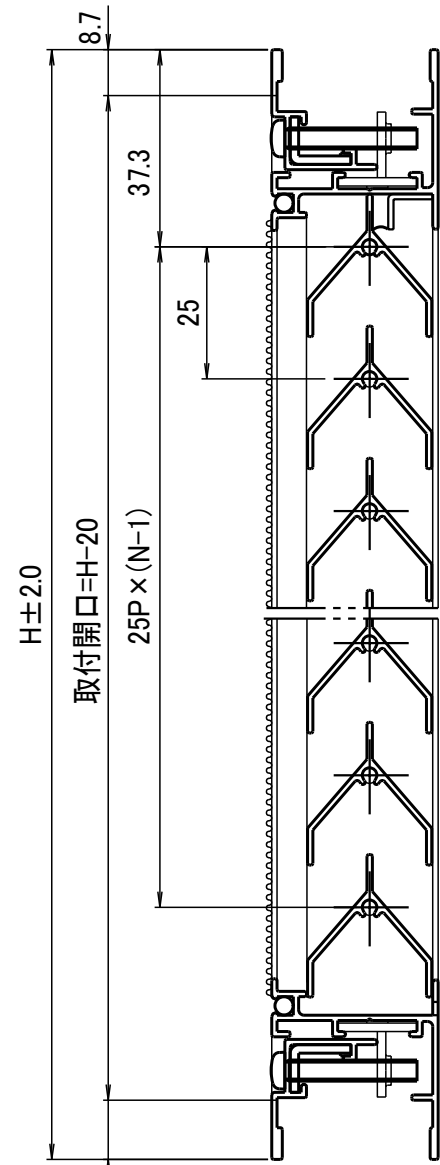
B-B断面図
