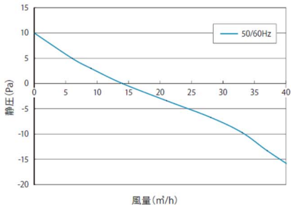
静圧-風量特性グラフ(P-Q曲線)
