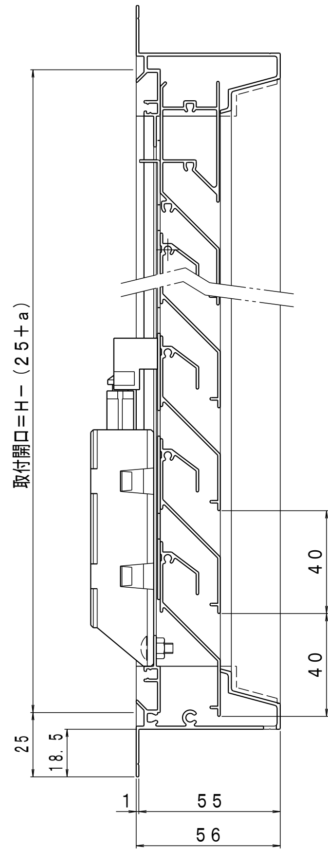
A-A断面図
