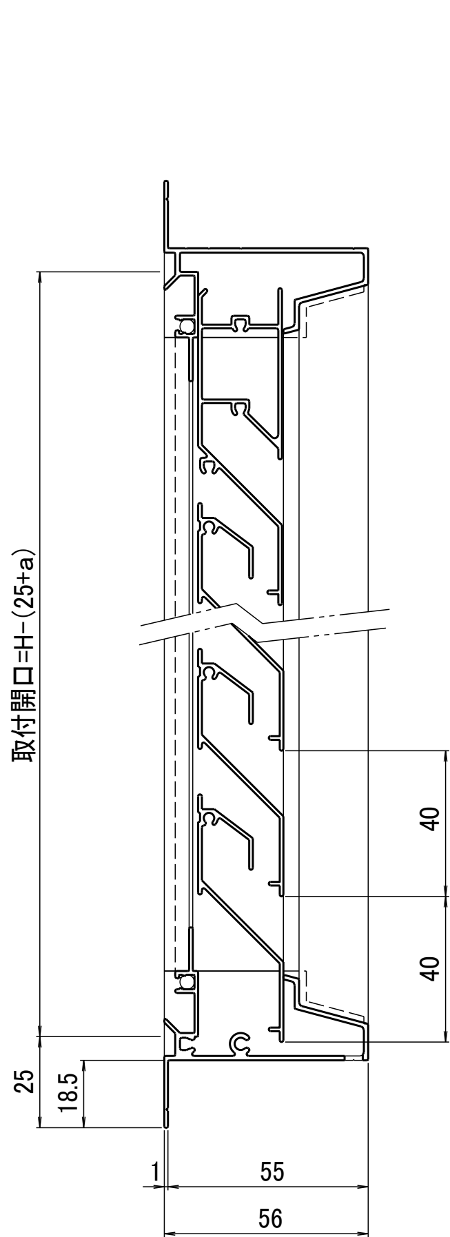
A-A断面図
