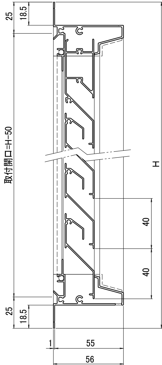
A-A断面図
