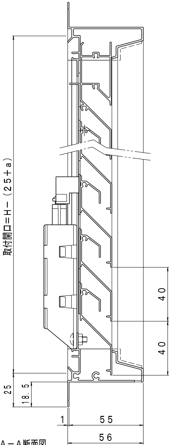
A-A断面図
