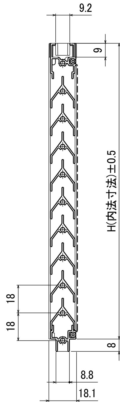
A-A断面図
