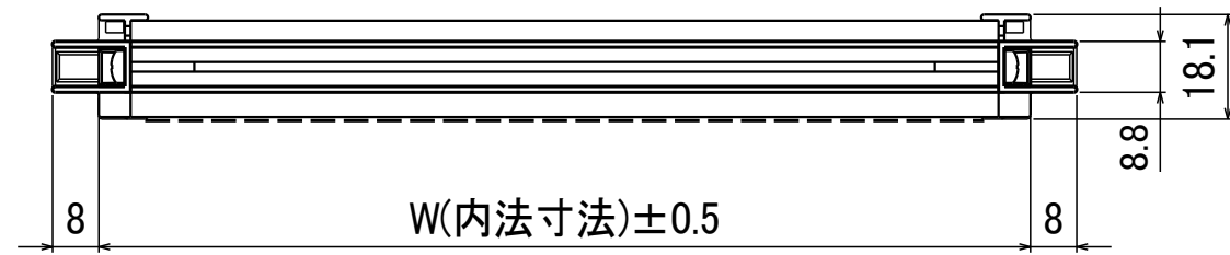
内観図
