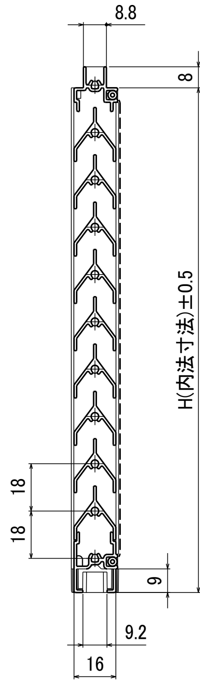
A-A断面図
