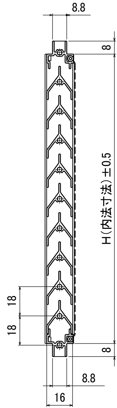
A-A断面図
