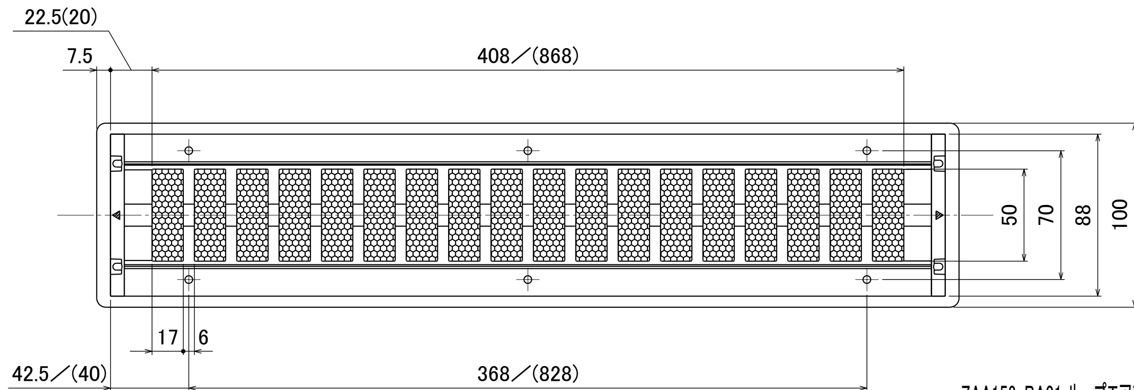
ZAA153-BA01 ループエアスリット(固定式) 商品図
