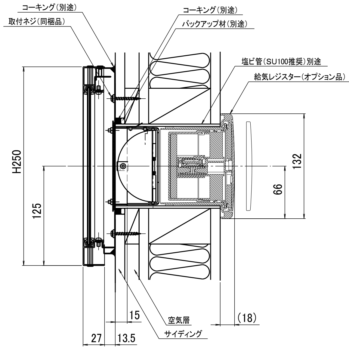
給気口(第三種換気)施工例
