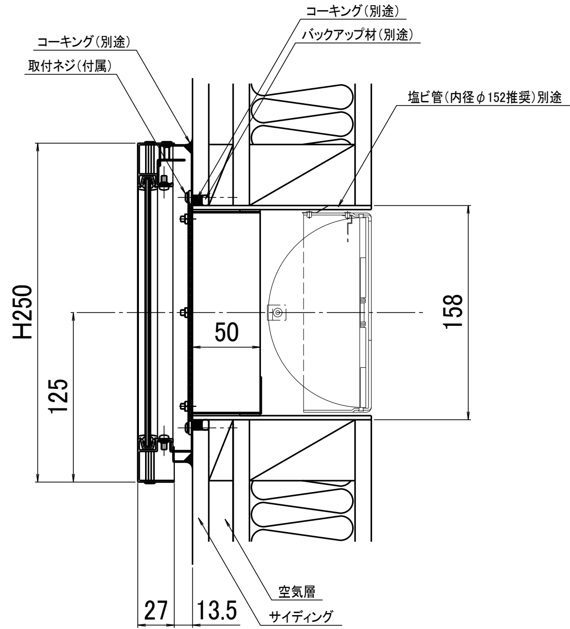
木造住宅小屋裏換気施工例
