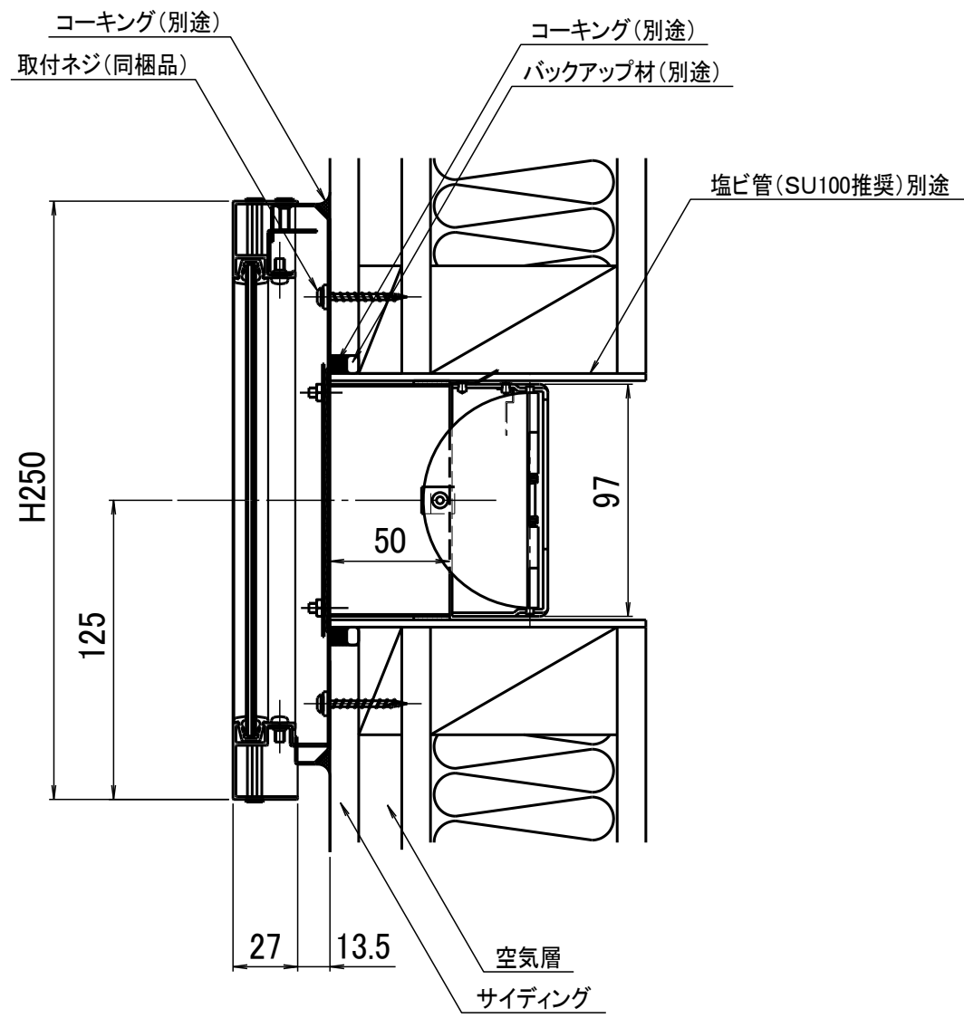
木造住宅小屋裏換気施工例
