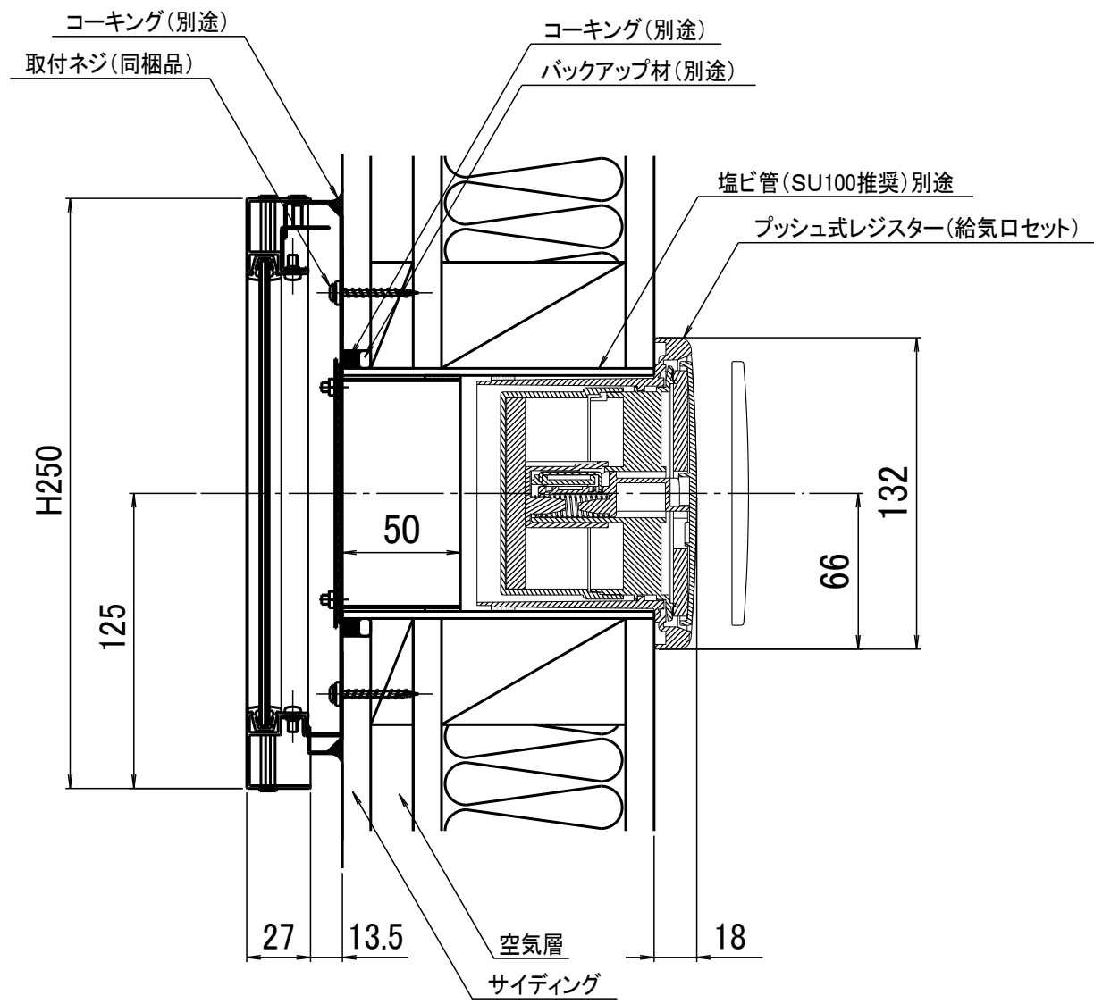
給気口(第三種換気設備)施工例
