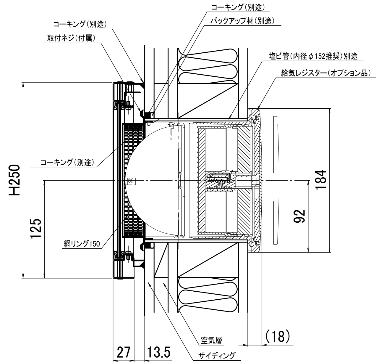
給気口(第三種換気)施工例
