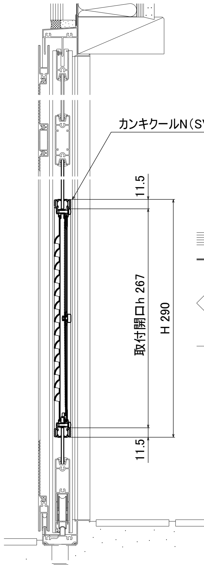
縦断面図
