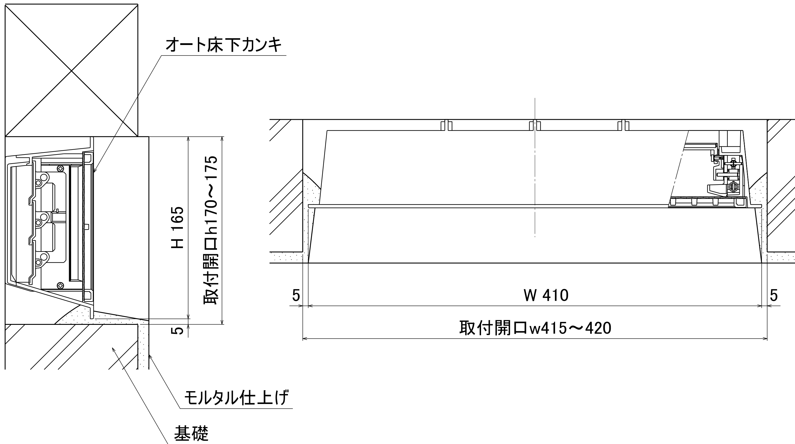
ZAA007-BA01 C オート床下カンキ 納まり図
