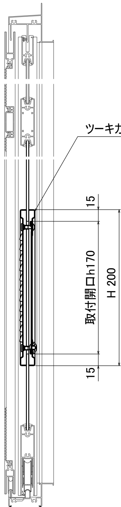
縦断面図
