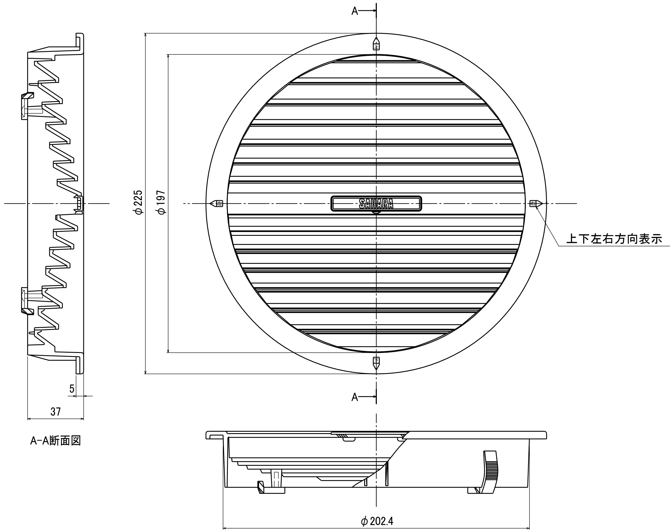
ZAA001-BA01-1 丸型床下換気ガラリ R1(常時開放)商品図
