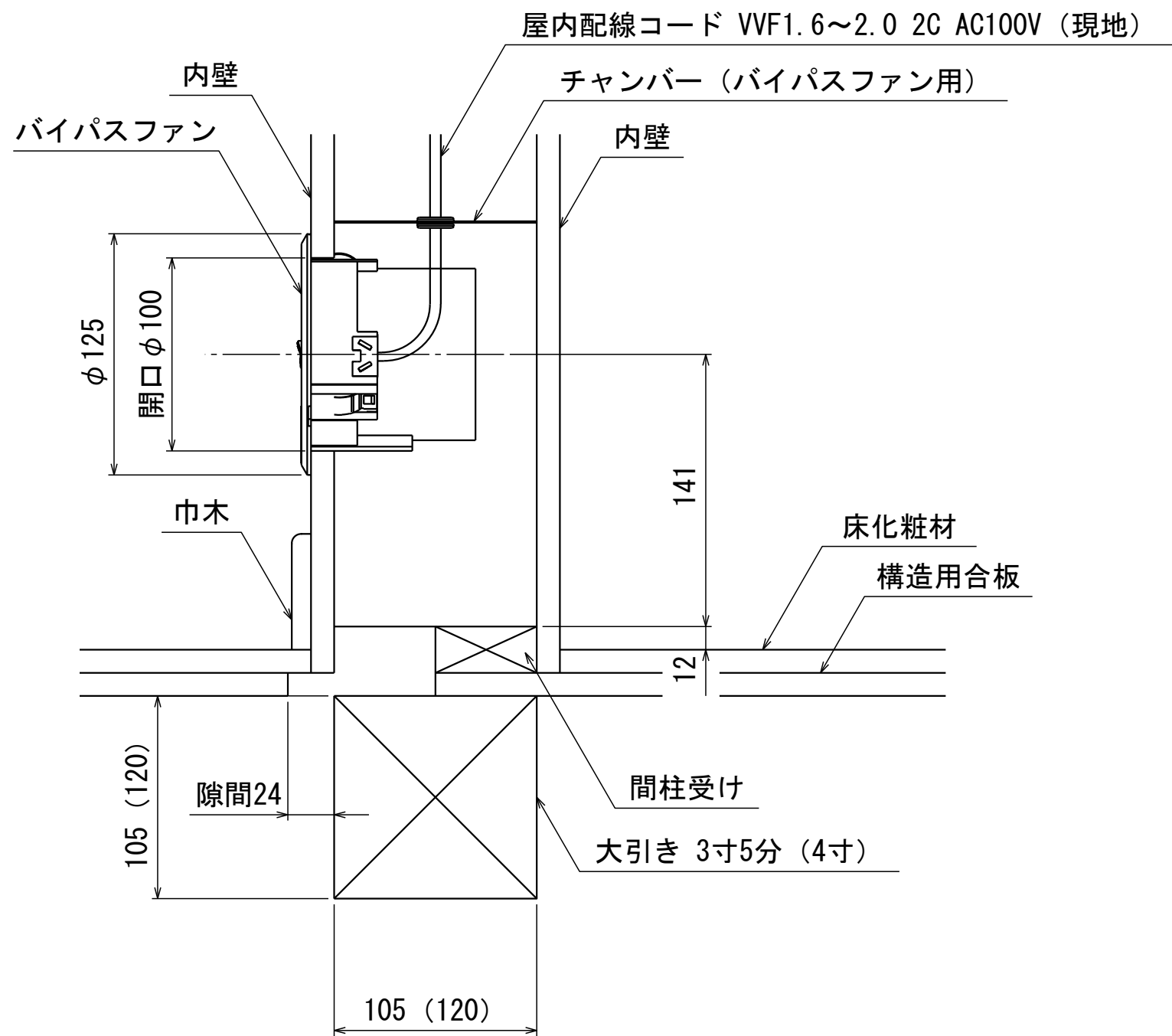
バイパスファン (排出側) 納まり図
