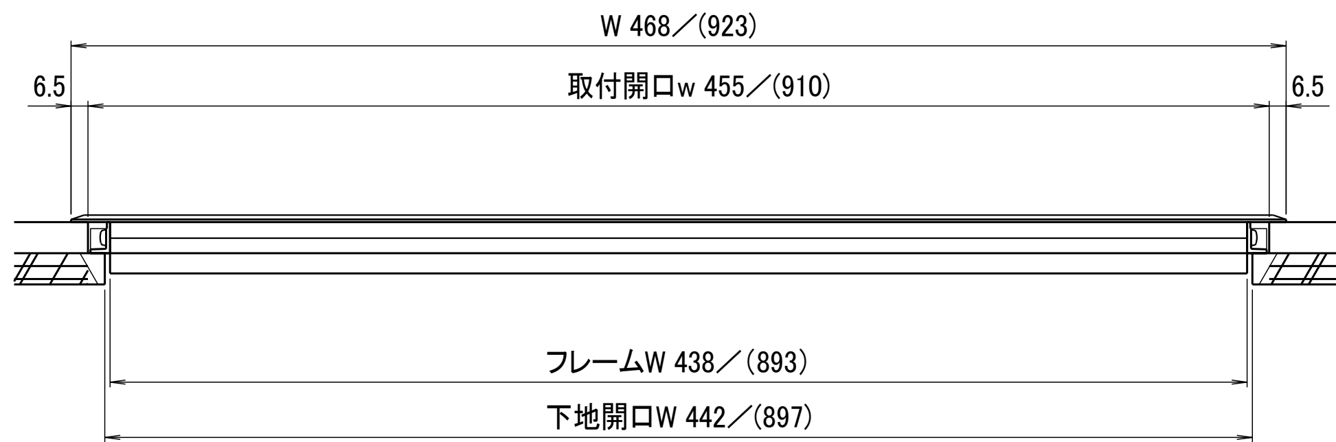
縦断面図
