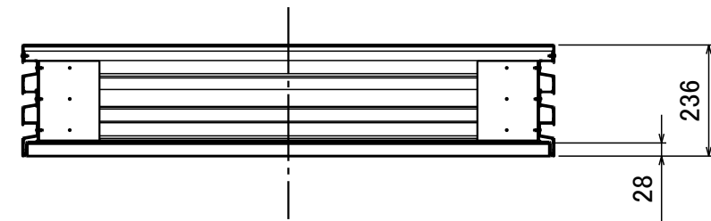
B-B断面图
