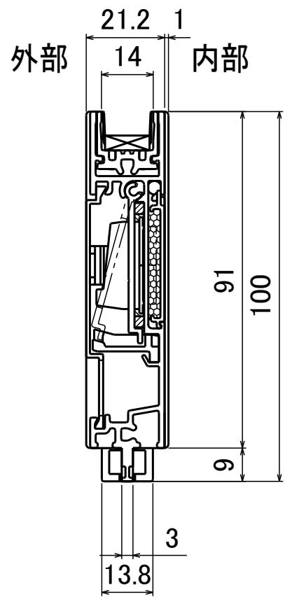
A-A断面図
