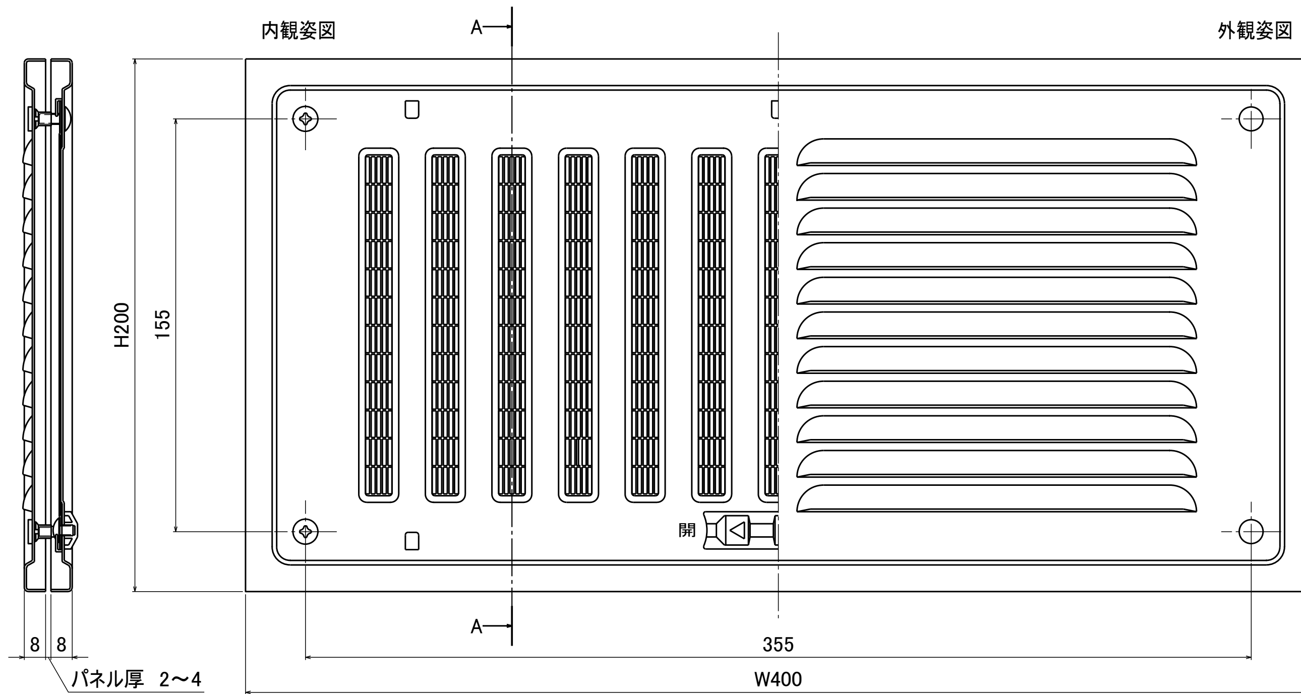
A-A断面図
