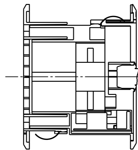
B-B断面図
