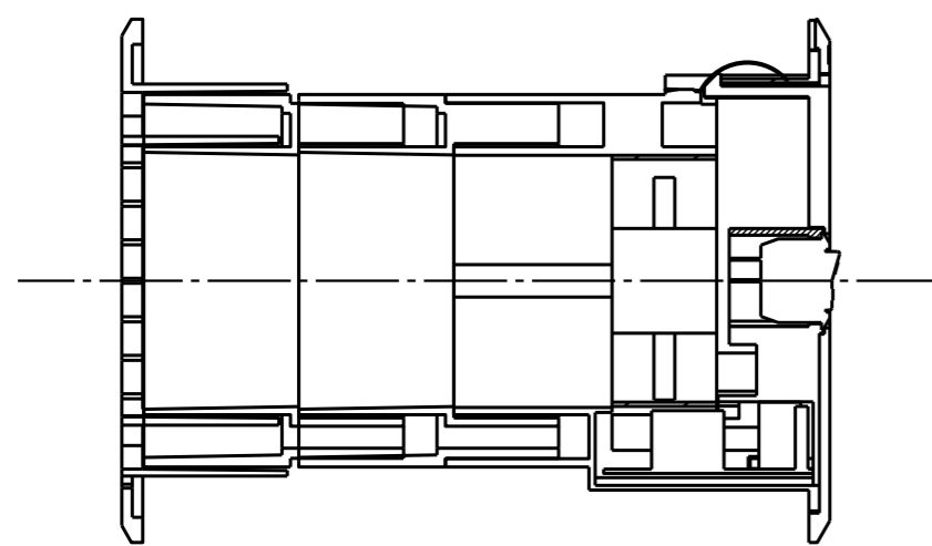
B-B断面図
