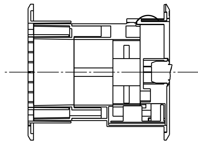
B-B断面図(アジャストリンク使用時)
