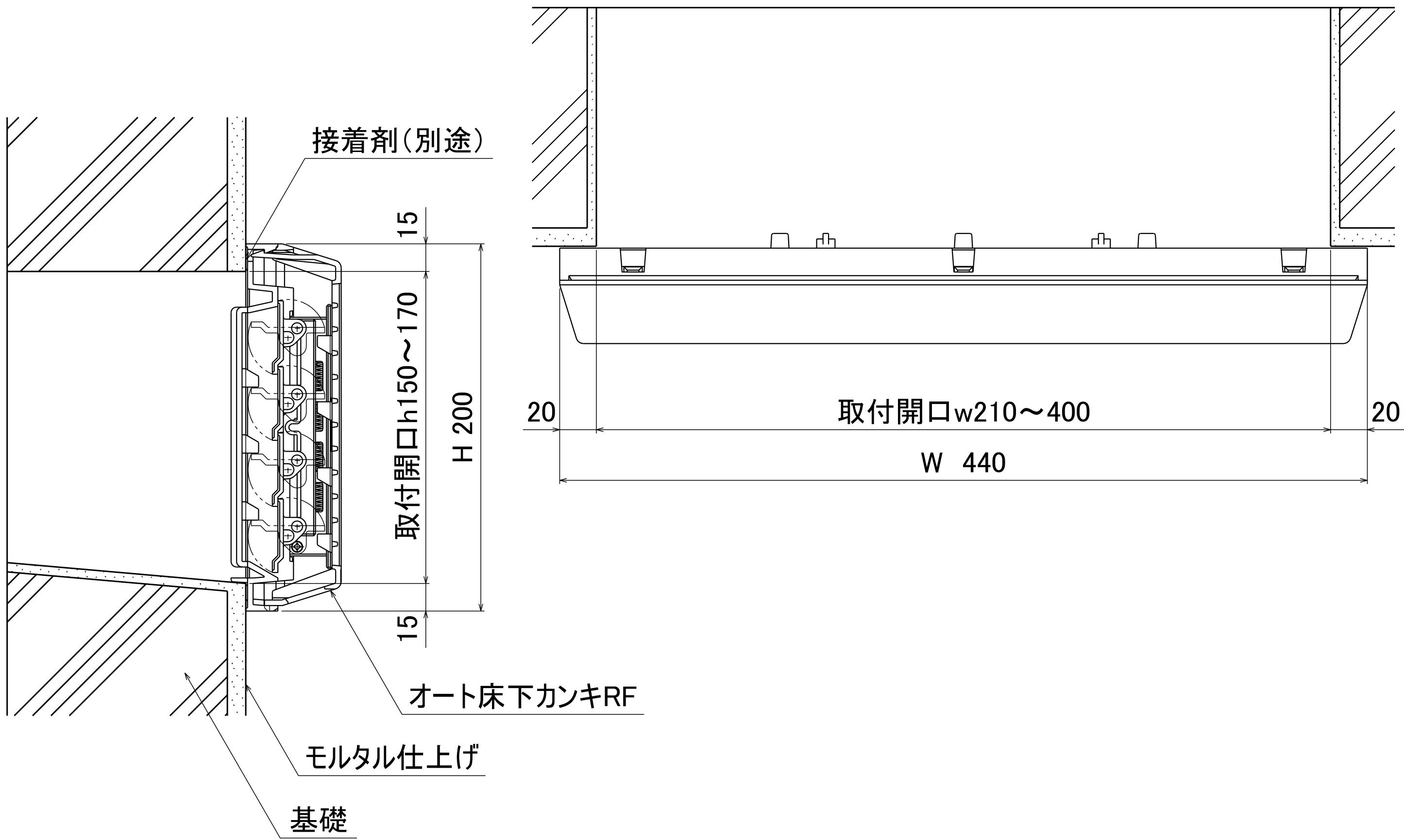
ZAA146-BA01 C オート床下カンキRF 納まり図
