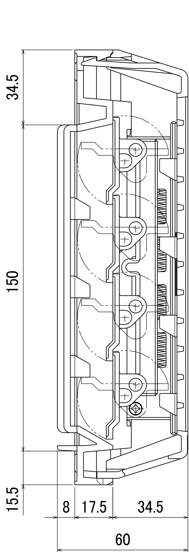
A-A断面図
