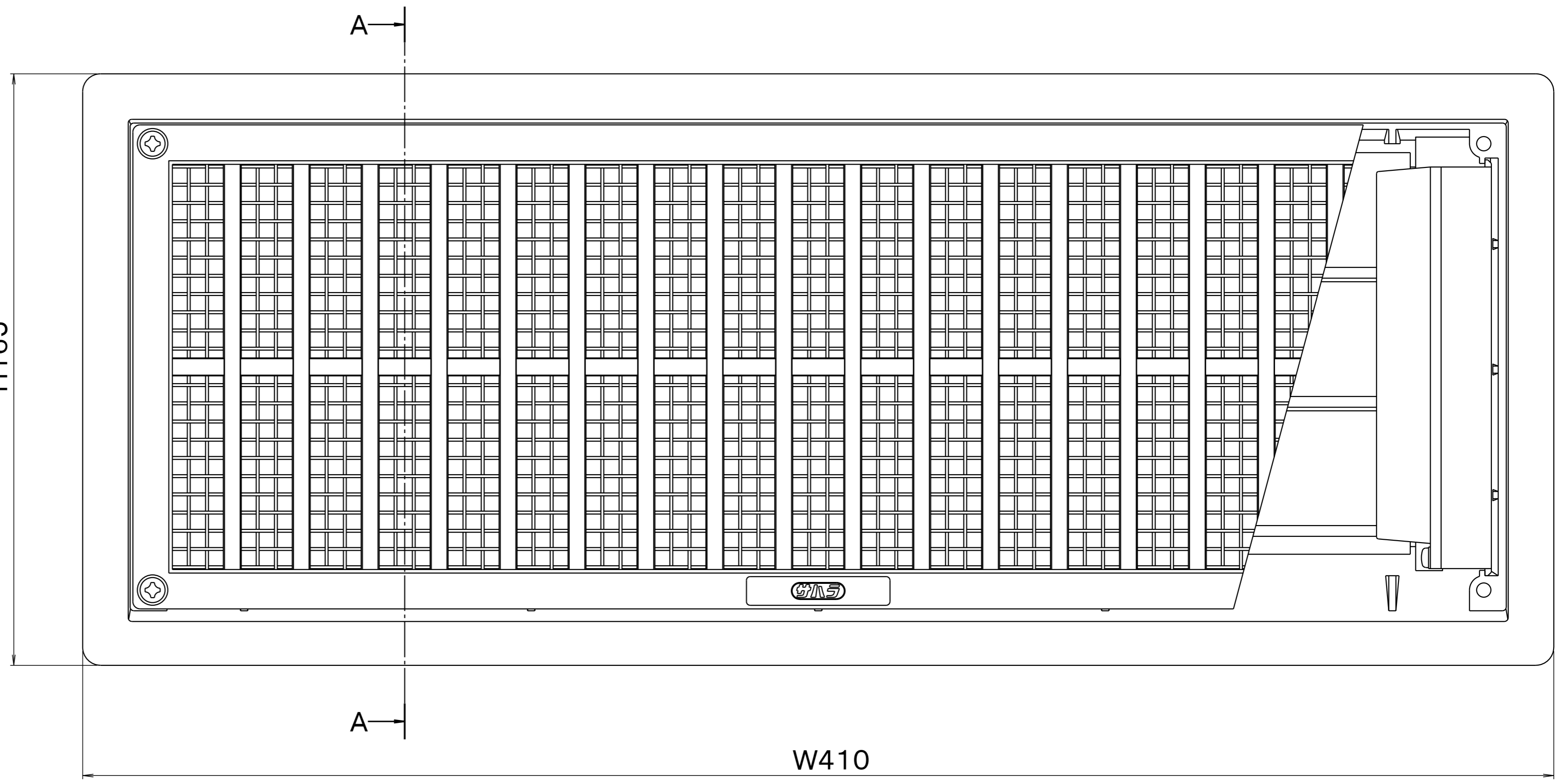
ZAA007-BA01 オート床下カンキ 商品図
