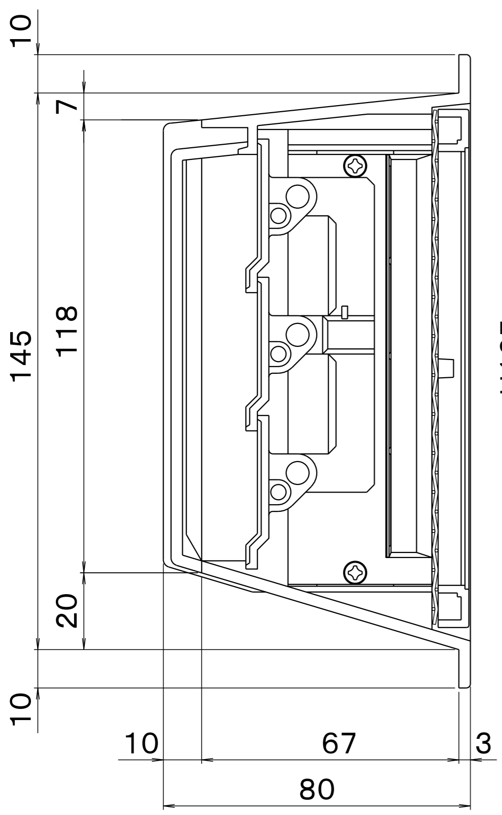
A-A断面図
