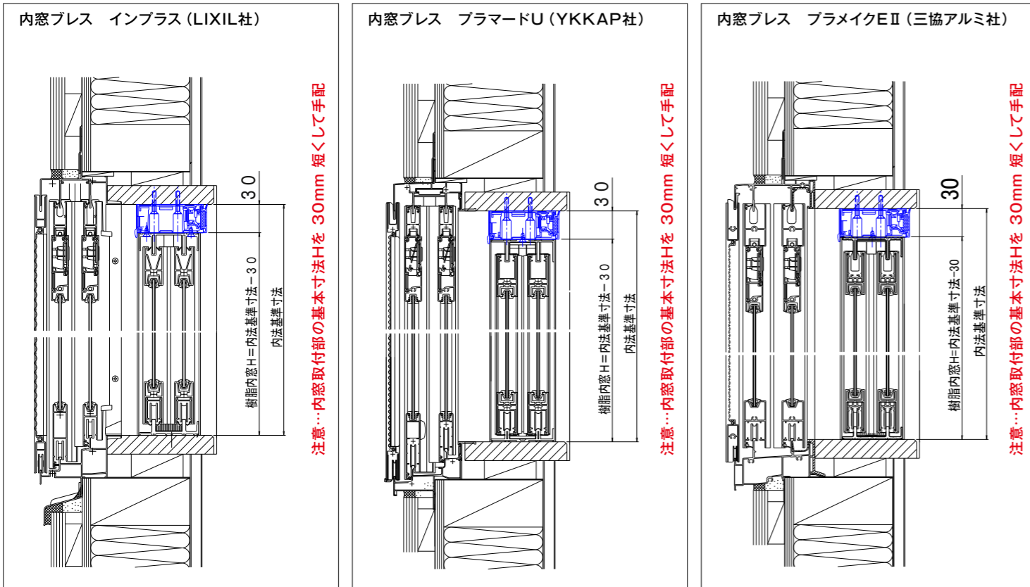
内窓ブレスの納まり図 (DXF・DWG・PDF) は、ホームページからダウンロードできます。
