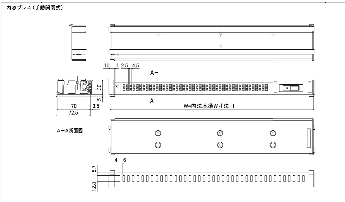
内窓ブレスの商品図 (DXF・DWG・PDF) は、ホームページからダウンロードできます。
