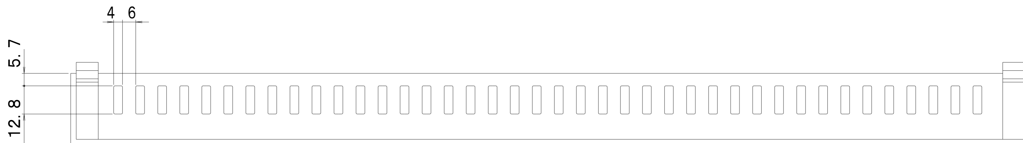
ZAA161-BA02 内窓プレス(手動開閉式)商品図
