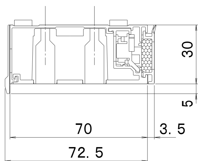
A-A断面図
