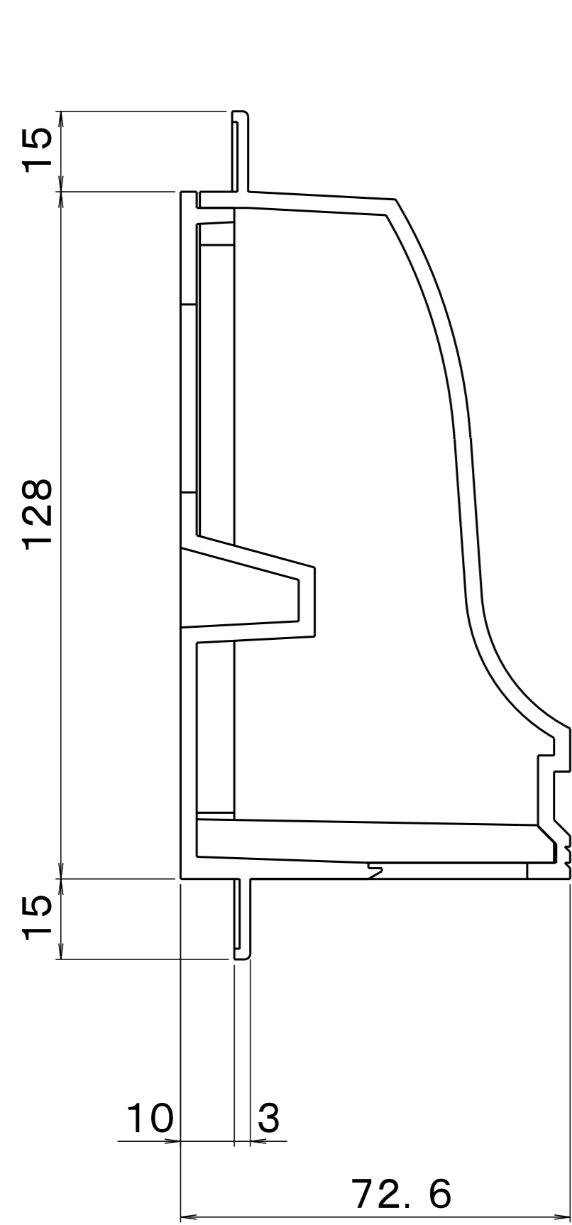
A-A断面図
