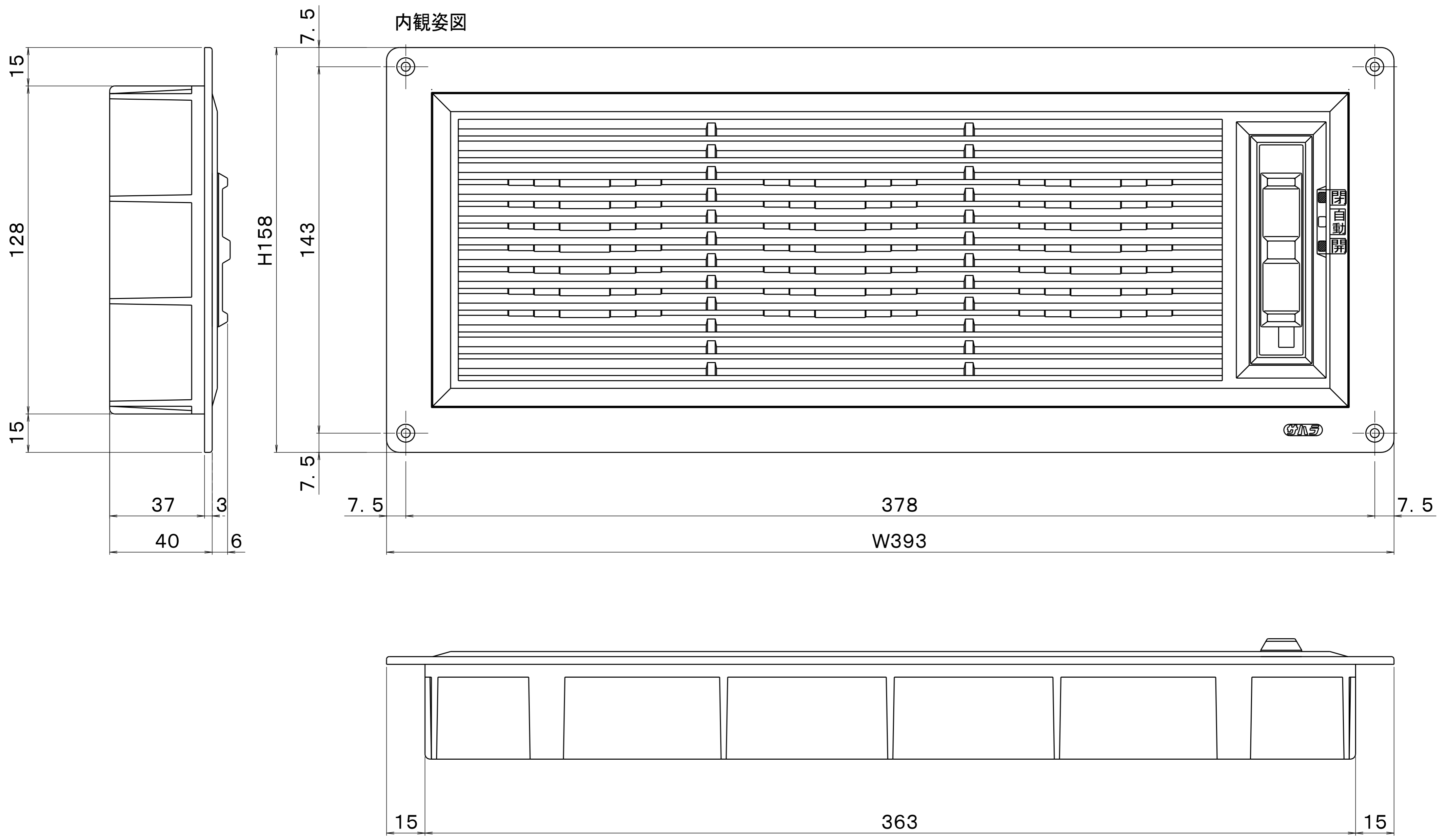
ZAA105-BA01A 快テキオートカンキ 商品図
