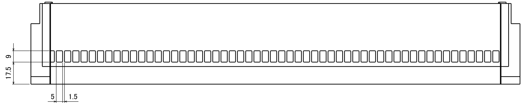
ZAA184-BB01 プロテクトプレス PW50G-26 商品図
