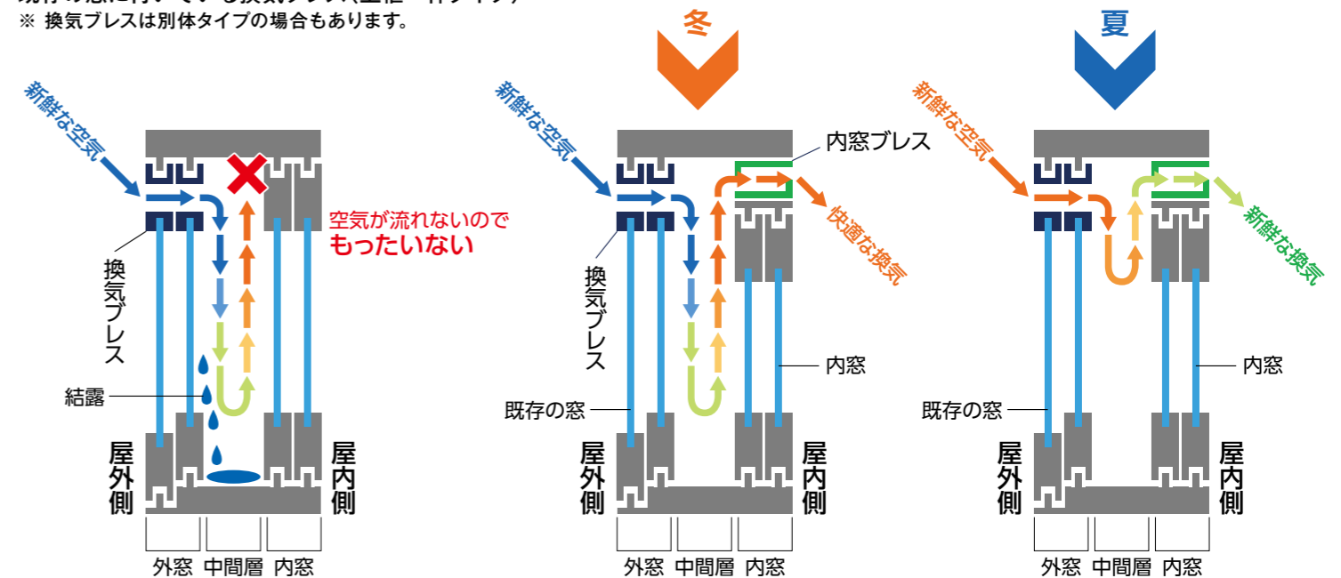
換気の機能を生かしていない 図-1 冬には快適な換気 図-2 夏にも計画的に換気 図-3 内窓に通気経路がないので空気が流れない 外窓と内窓の空間に空気の流れをつくることで断熱と換気が両立できる
