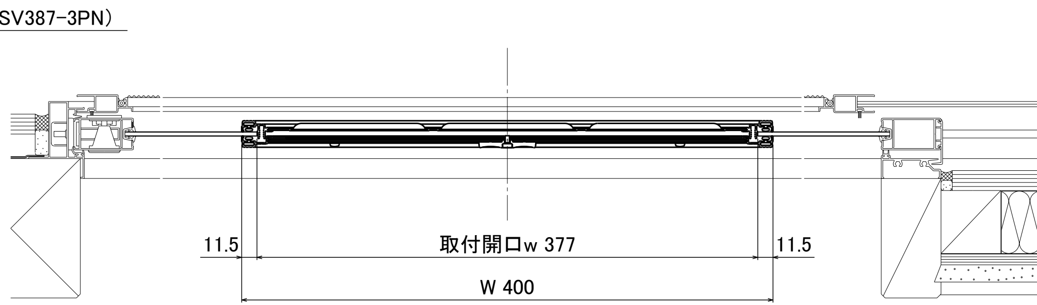
横断面図
